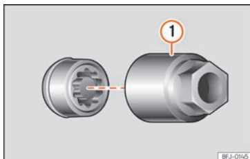
Rys. 42 Śruba przeciwwkradzieżowa do koła z nasadką i adapterem.
