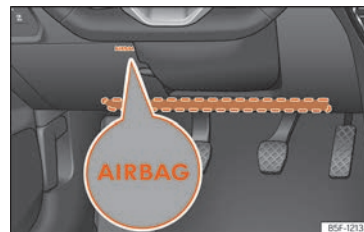
Rys. 22 Po stronie kierowcy: umiejscowienie kolanowej poduszki powietrznej
