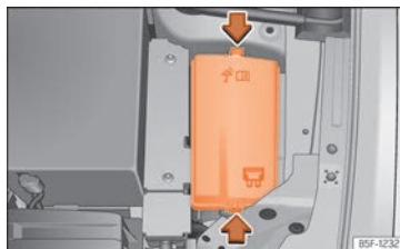
Rys. 56 W komorze silnika: pokrywa skrzynki bezpieczników.
