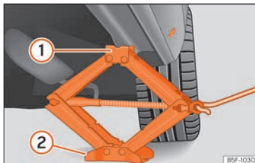
Rys. 46 Belka poprzeczna: podstawianie podnośnika pod pojazd.
