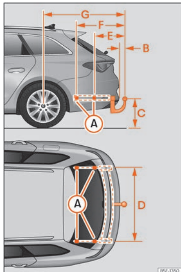
Rys. 207 Punkty graniczne i punkty mocowania haka holowniczego.
