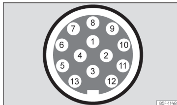
Rys. 205 Schemat: opis styków w gnieździe elektrycznym przyczepy.
