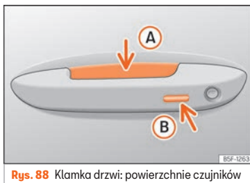
Rys. 88 Klamka drzwi: powierzchnie czujników
