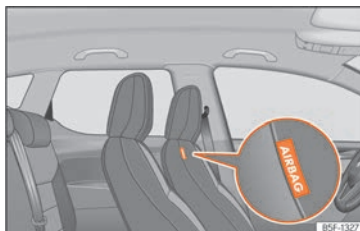
Rys. 24 W wewnętrznym obiciu oparcia siedzenia kierowcy: środkowa poduszka powietrzna.
