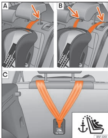
Rys. 34 Siedzenia tylne: regulacja i montaż paska Top Tether.
