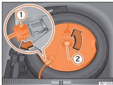
Rys. 239 W bagażniku: wyjąć głośnik niskotonowy.
