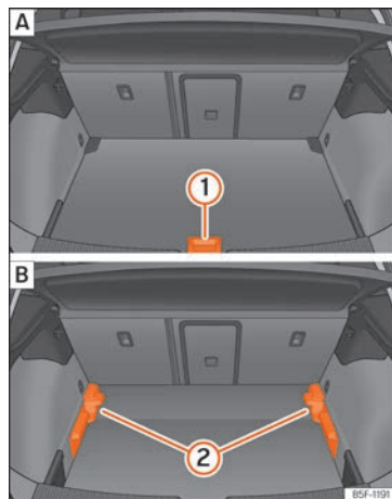
Rys. 129 Regulowana podłoga bagażnika: A pozycja uniesiona; B pozycja obniżona.
