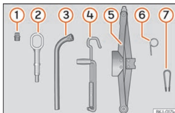
Rys. 38 Pod płytą podłogi w bagażniku: zestaw narzędzi samochodowych.
