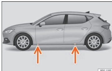
Rys. 45 Punkty unoszenia.
