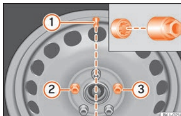
Rys. 44 Zmiana koła: zawór opony ① oraz prawidłowe położenie śruby zabezpieczającej przed kradzieżą koła ② lub ③.
