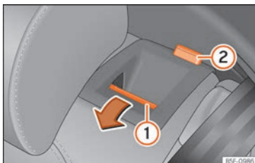
Rys. 118 Tyłne siedzenie: składanie oparcia.
