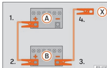
Rys. 49 Schemat połączeń dla pojazdów bez systemu Start-Stop.
