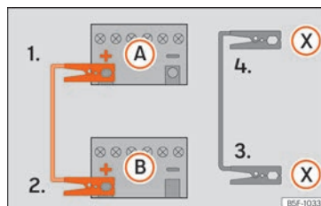
Rys. 50 Schemat połączeń dla pojazdów z systemem Start-Stop.
