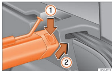
Rys. 139 W bagażniku: zdejmowanie siatki dzielącej.
